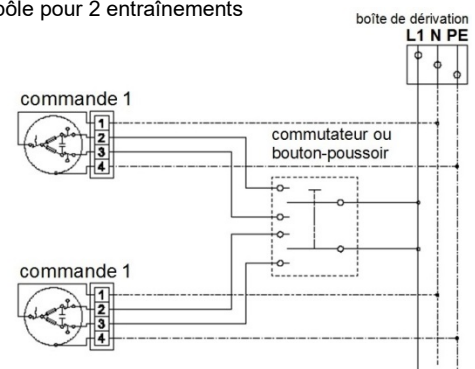
Schéma de connexion, commutateur / bouton-poussoir 1-pôle
