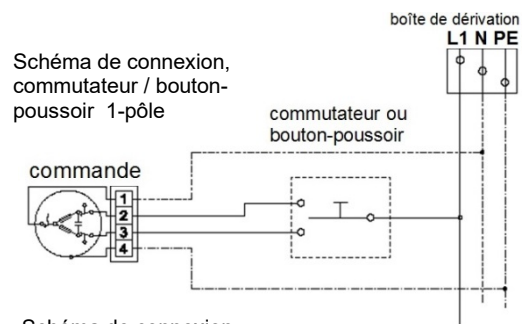
Schéma de connexion, commutateur / bouton-poussoir 1-pôle
